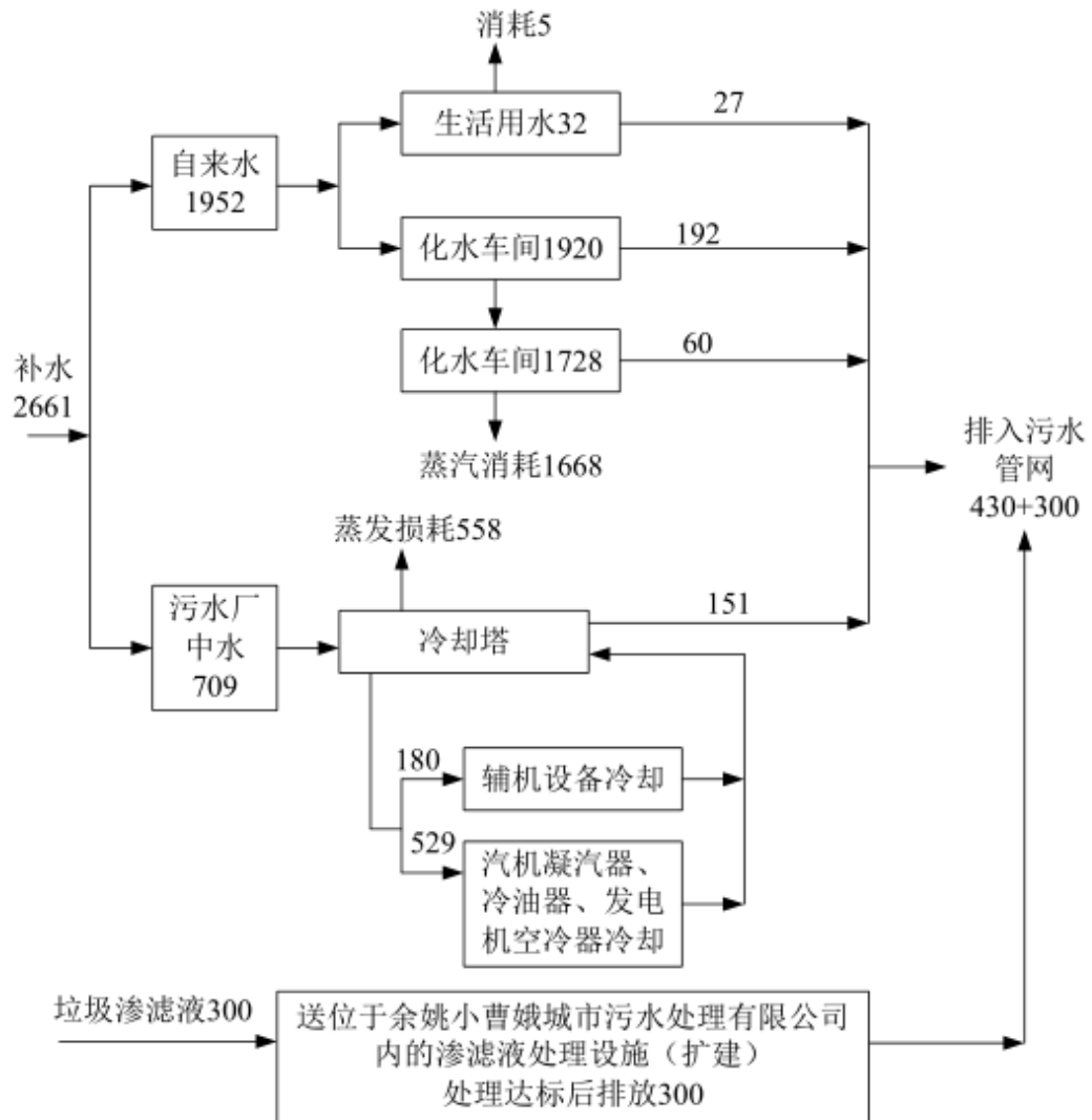
图4-2冷却排污水纳管、生活污水、化水废水、其他生产及生活废水工艺图
